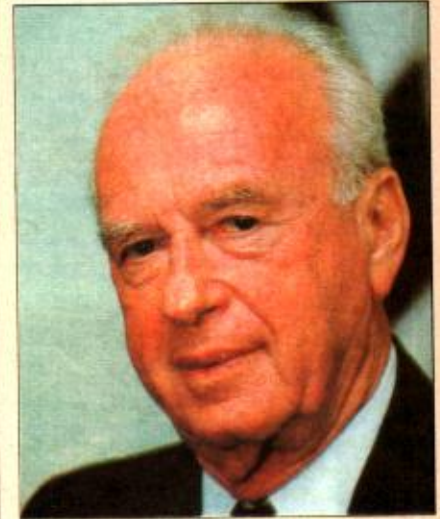
رابين
