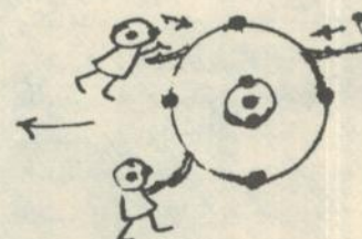
وسط ذرة من النيوتروجين تبيع لها ثتها الايكترونية الارتباط بثلاث من الايدروجين .
