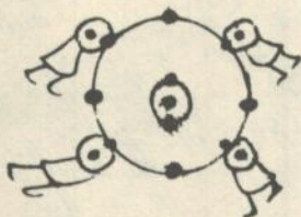
وعندما يتزوج الكربون بالاربعة يصبح على هيئة جزيء غاز
