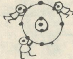
فترتبط بها عن طريق اليكترون ويتحول الجميع الى نشادر
